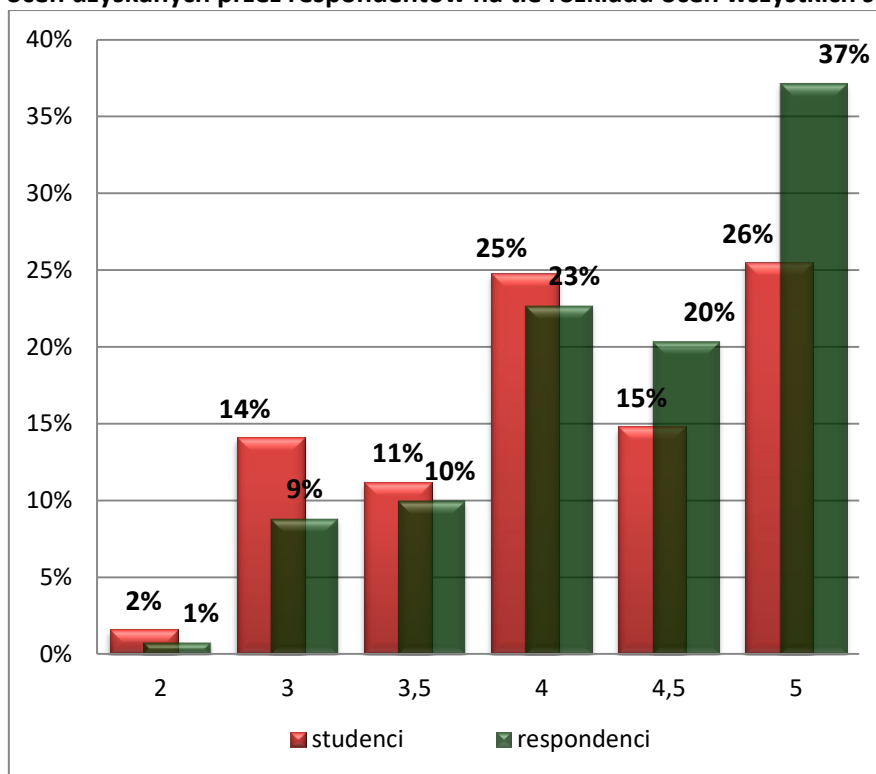
Rozkład ocen uzyskanych przez respondentów na tle rozkładu ocen wszystkich studentów
